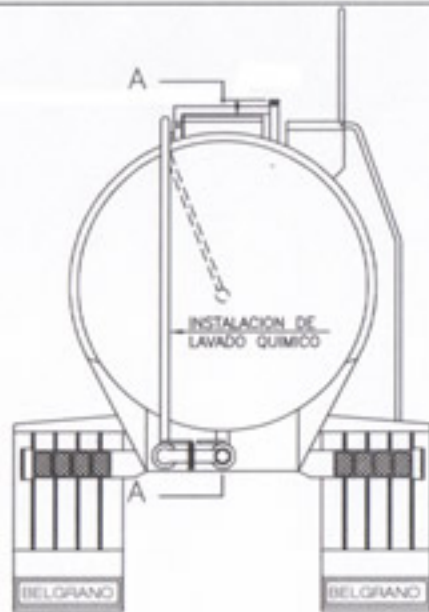
VISTA TRASERA
